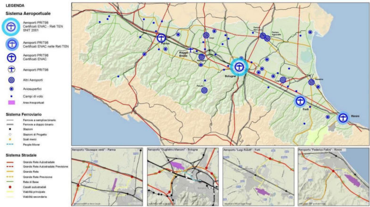
Figura 3-5 Dettaglio del sistema aeroportuale, ferroviario e stradale.
