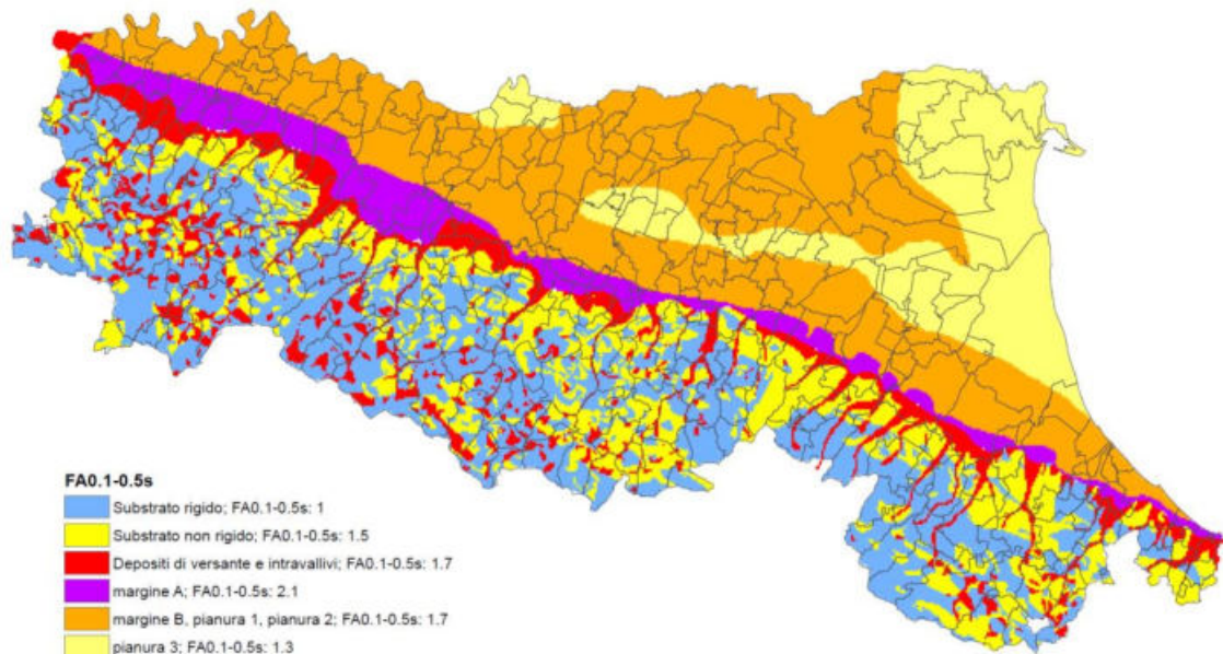
Figura 2-12 Mappa dei fattori di amplificazione in accelerazione per periodi T compresi tra 0,1 s e 0,5 s ( FA_{0,1-0,5s} ).
