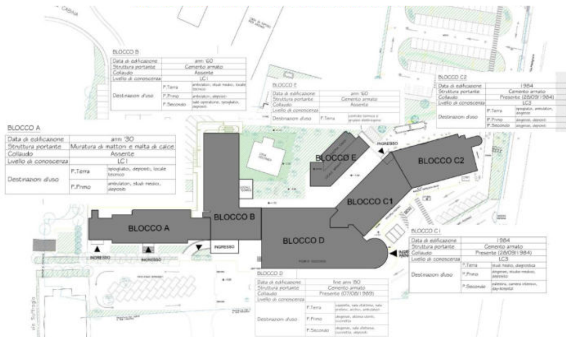
Figura 2-15 Rappresentazione schematica delle vulnerabilità strutturali nelle schede di verifica post sisma.
