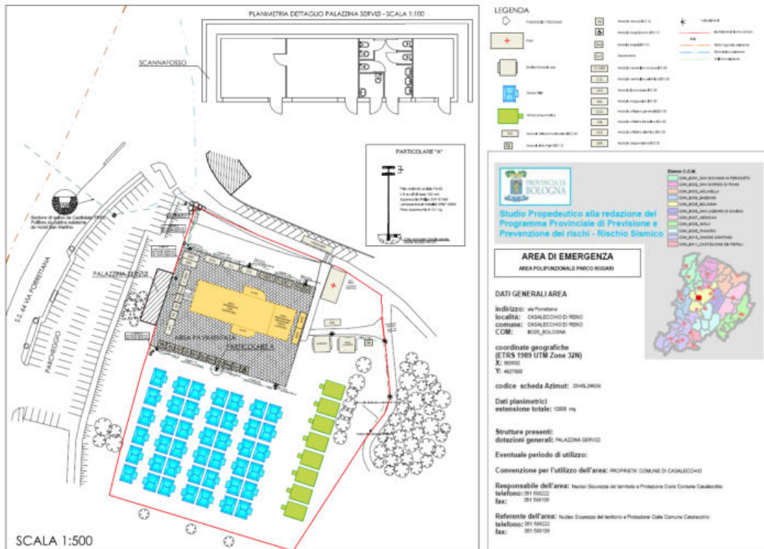
Figura 4-4 Schema rappresentativo dell'allestimento di un possibile campo di accoglienza.
