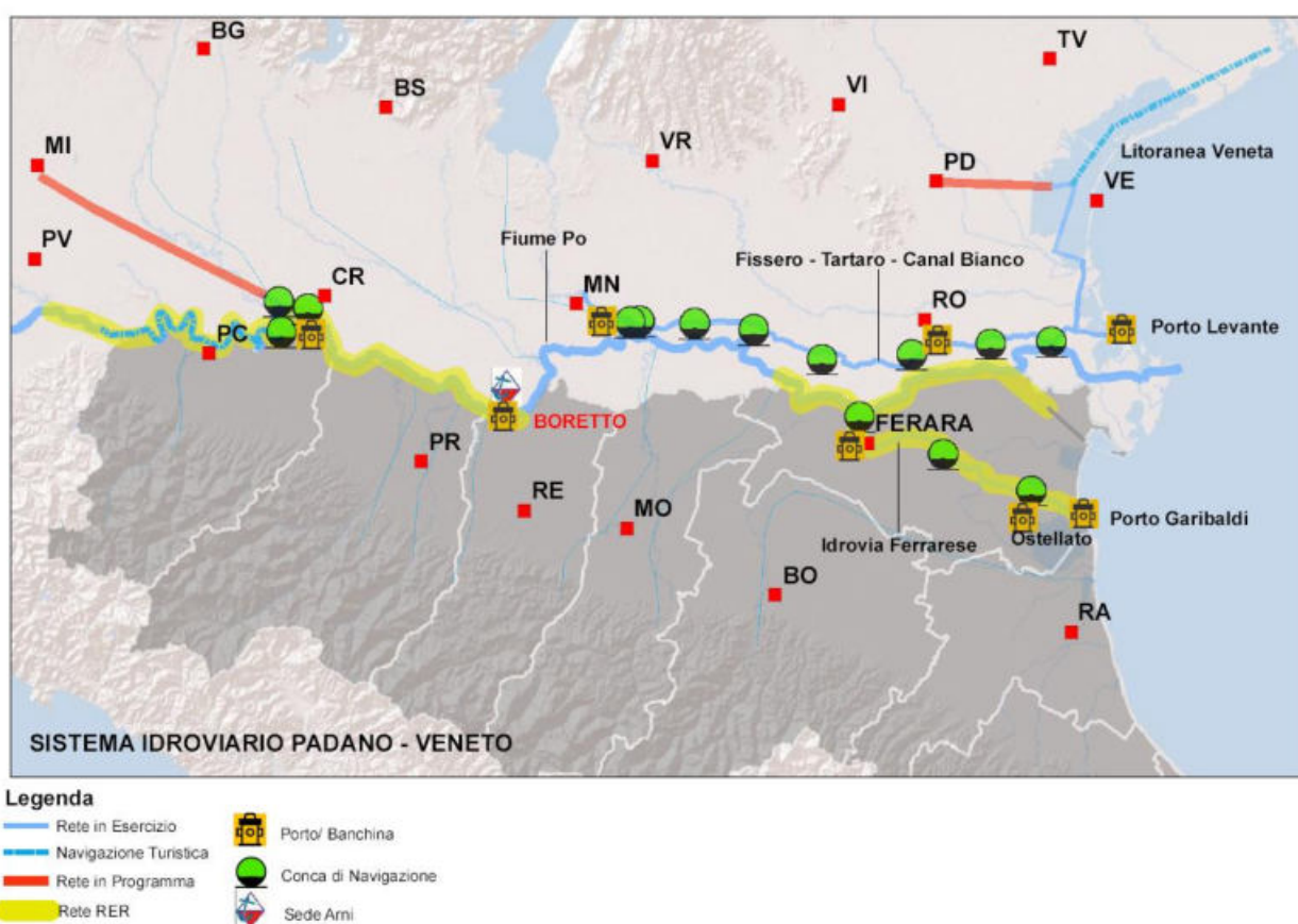
Figura 3-13 Sistema idroviario padano-veneto – Rete in esercizio.
