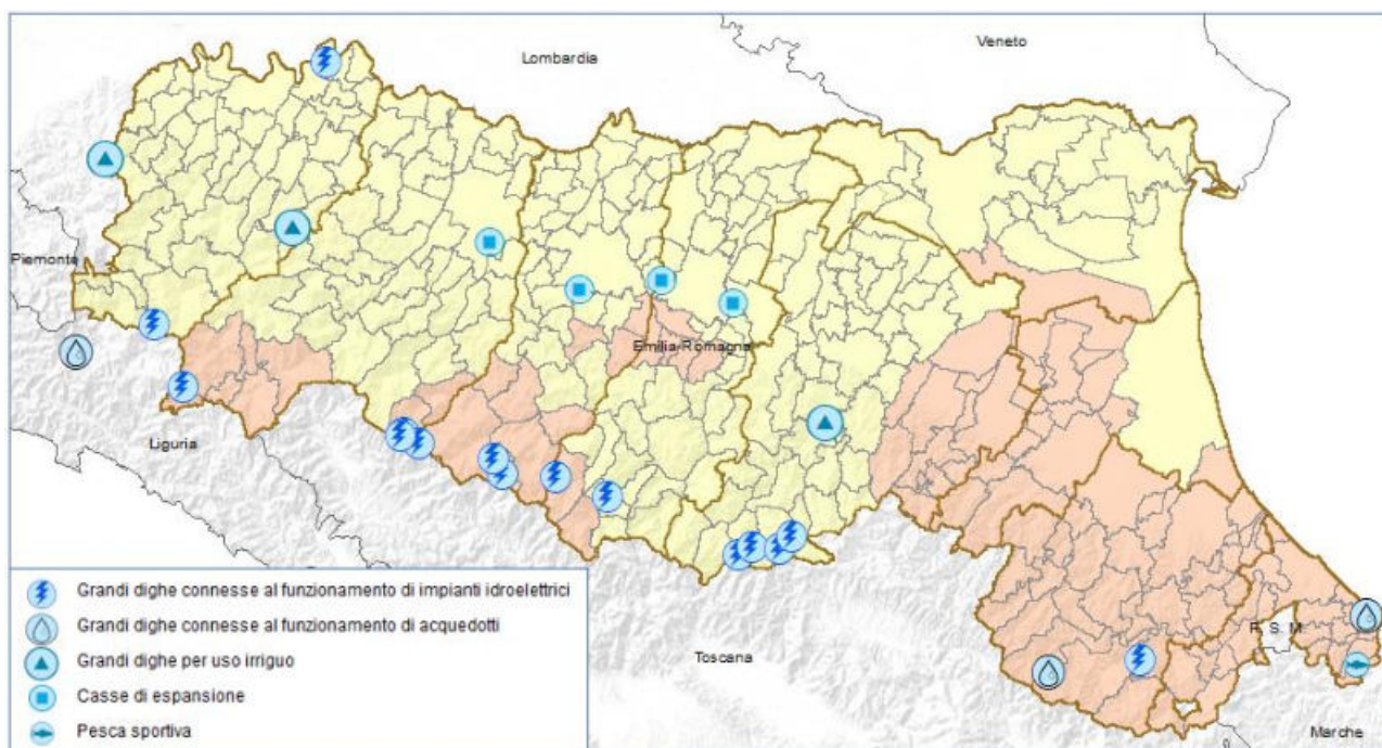
Figura 2-25 Distribuzione territoriale e classificazione delle grandi dighe (rappresentazione in Moka: Rischi ed effetti indotti).
