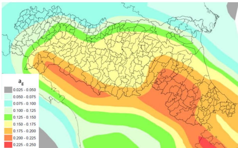
Figura 2-4 Mappa di pericolosità sismica di base MPS04 (OPCM 3519/2006) per l'Emilia-Romagna e aree limitrofe per T_R=475 anni.
