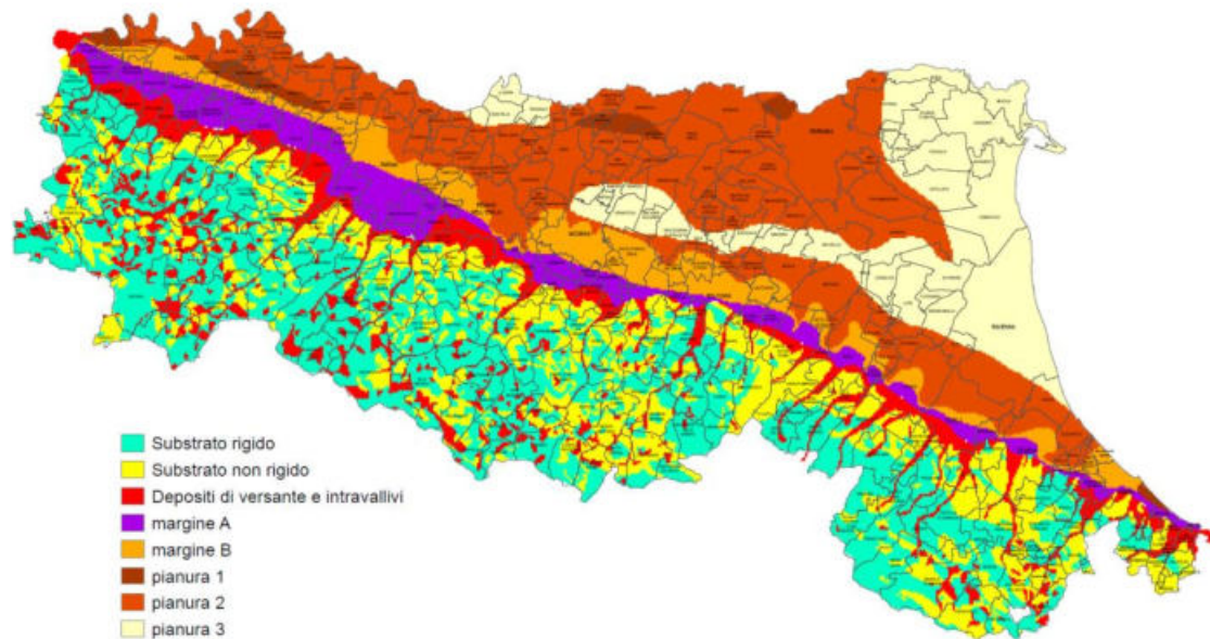
Figura 2-8 Macrozonazione regionale dei principali ambienti geologico-morfologici in prospettiva sismica.
