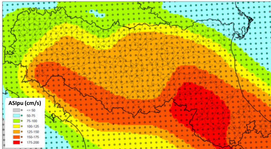
Figura 2-11 Mappa dei valori ASl_{PU} in Emilia-Romagna e aree limitrofe, T_R=475 anni.
