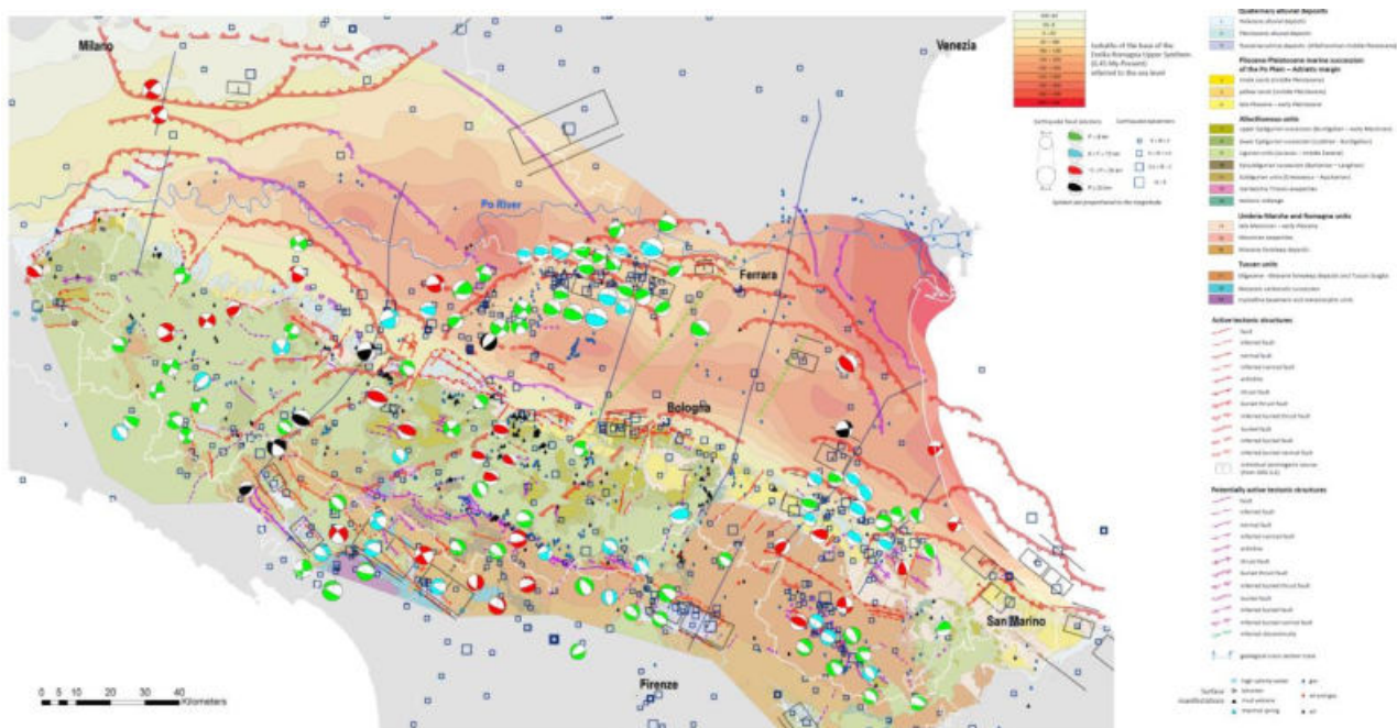
Figura 2-2 Schema sismotettonico dell'Emilia-Romagna e aree limitrofe (da Martelli et al., 2017).
