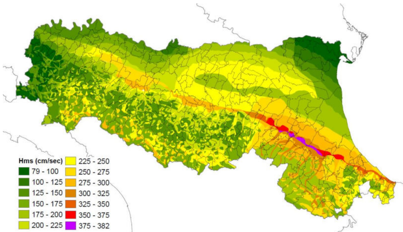
Figura 2-13 Mappa dei valori di H_{MS} (pericolosità sismica al sito per 0,1s \leq T \leq 0,5s e T_R=475 anni) in Emilia-Romagna.
