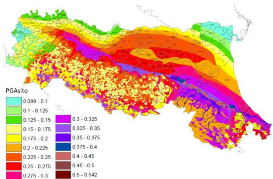
Figura 2-10 Macrozonazione sismica regionale in termini di PGA attesa al sito per T_R=475 anni.
